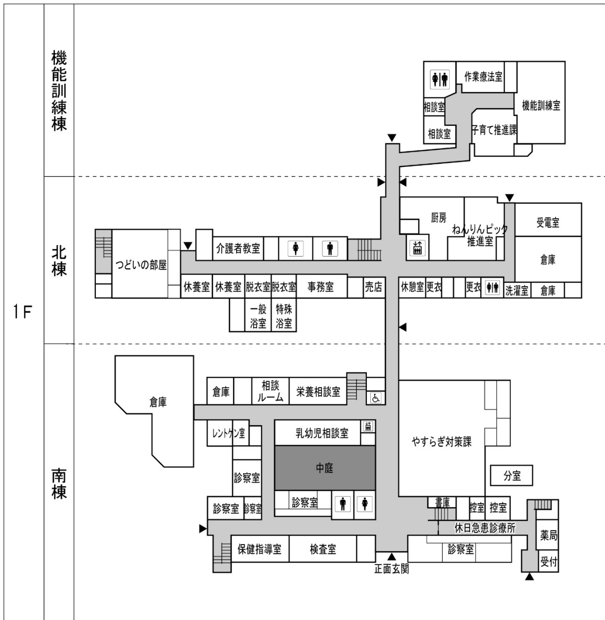
【市民総合センター 1F 平面図】
