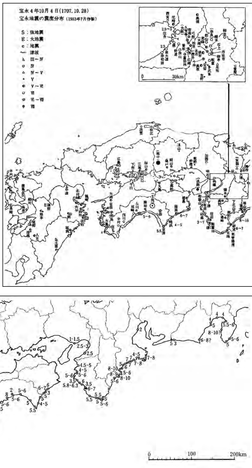
No.7 1707年 宝永地震(震度分布と津波波高)
