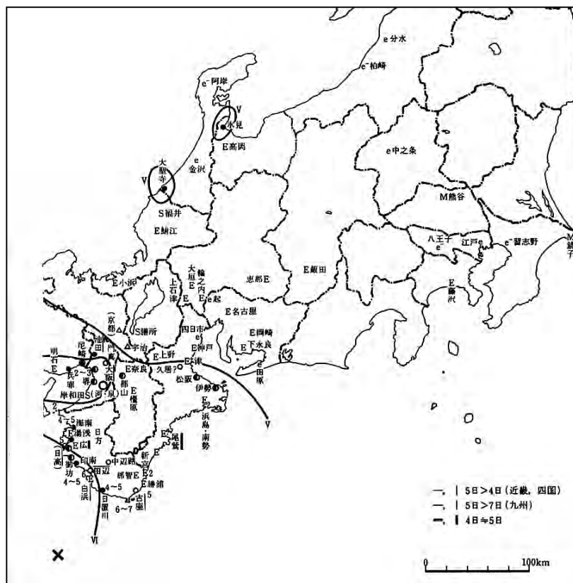
No.9 1854年 安政南海地震（震度分布）
