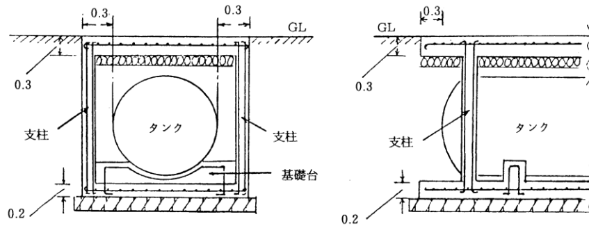
支柱により支える例（単位：m）
