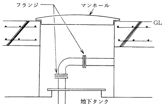
配管の接続例
