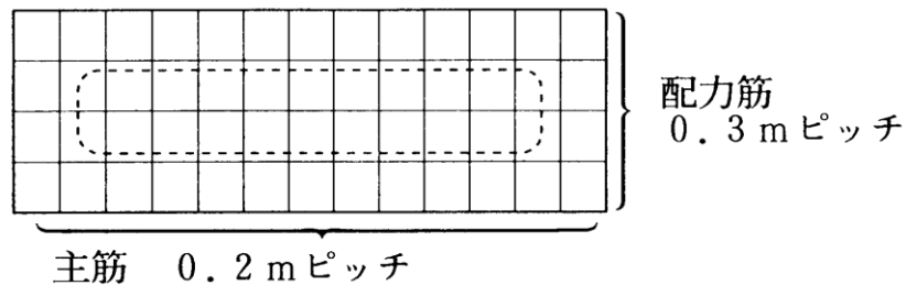
タンクふたの配筋例
