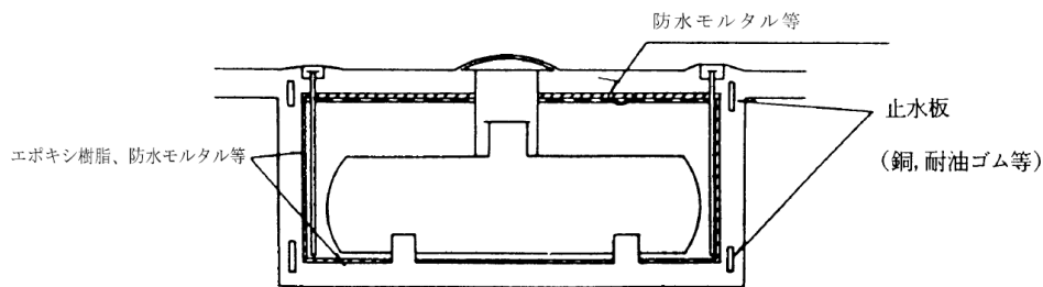
タンク室の防水措置の例
