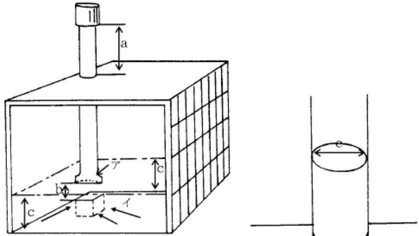
例図1 ーためますを整備室の隅に設ける場合の例ー
