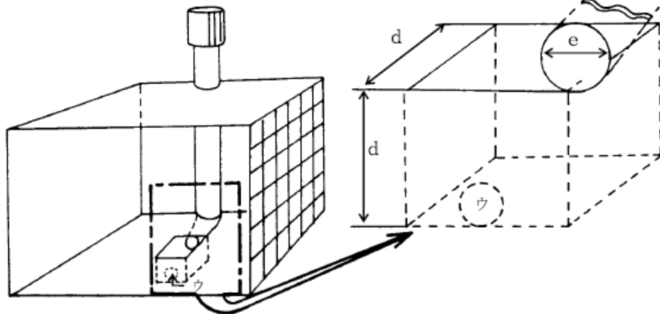
例図2 ーためますを整備室の中央に設ける場合の例ー
